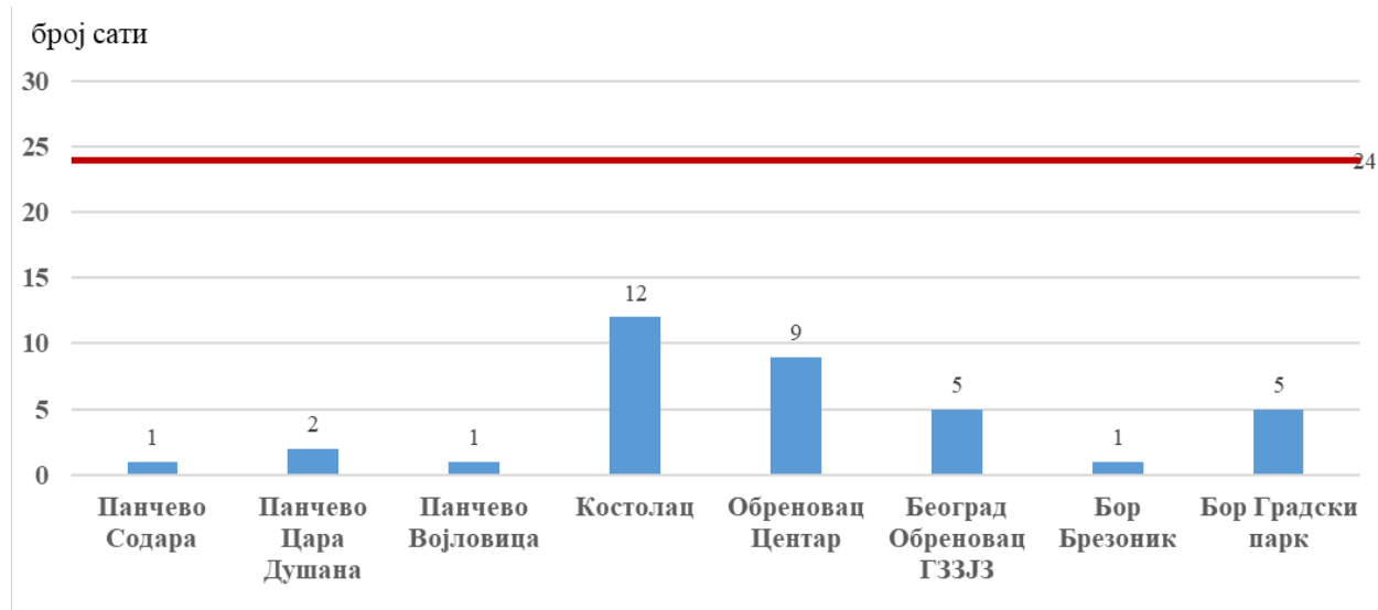
Слика 3.1.5. Мерна места у Републици Србији током 2023. године на којима је регистровано прекорачење сатне граничне вредности сумпор диоксида
