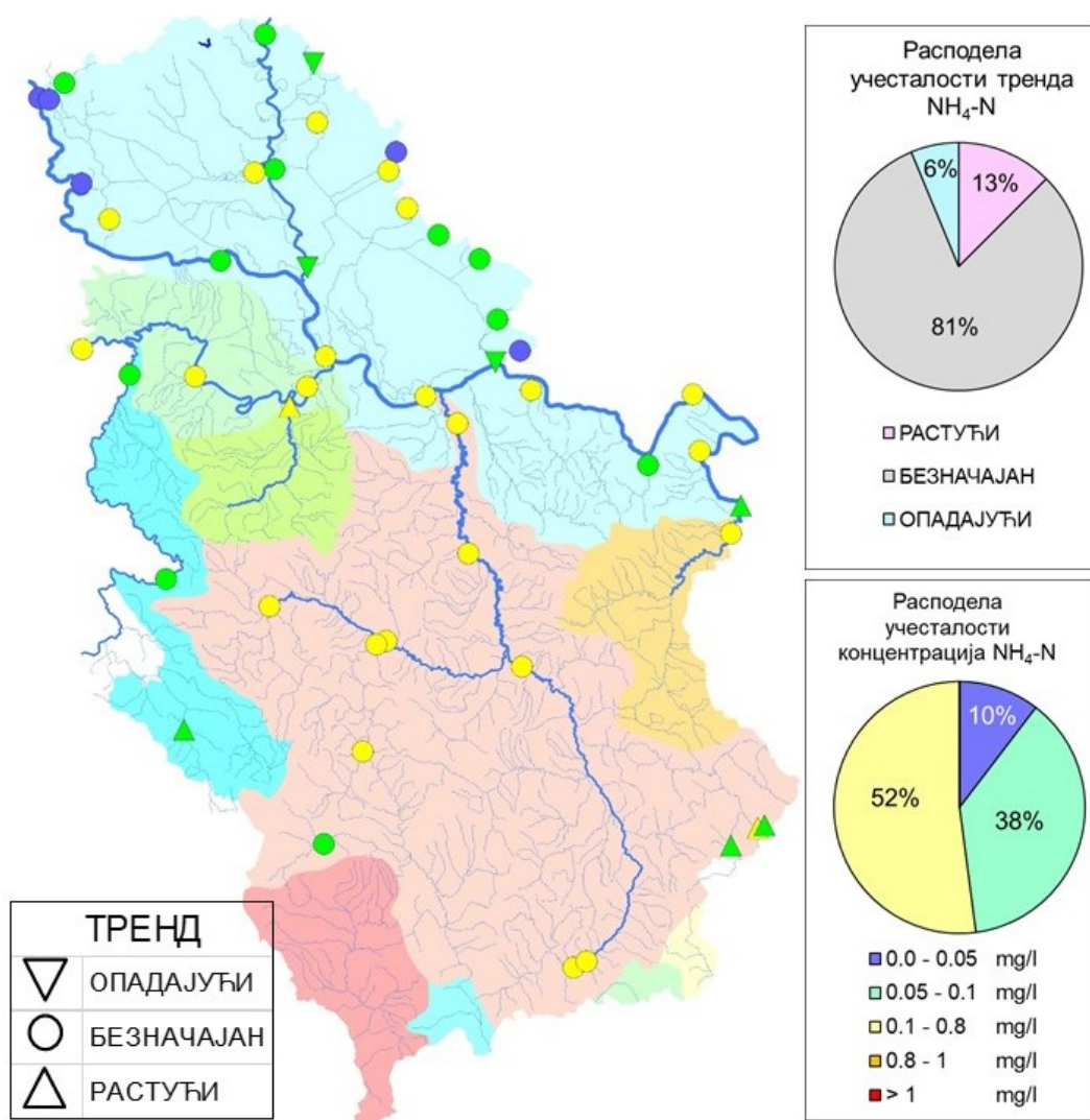
Слика 3.1.35. Тренд и средња вредност концентрација амонијума у водотоцима Републике Србије (2013-2022. године)
