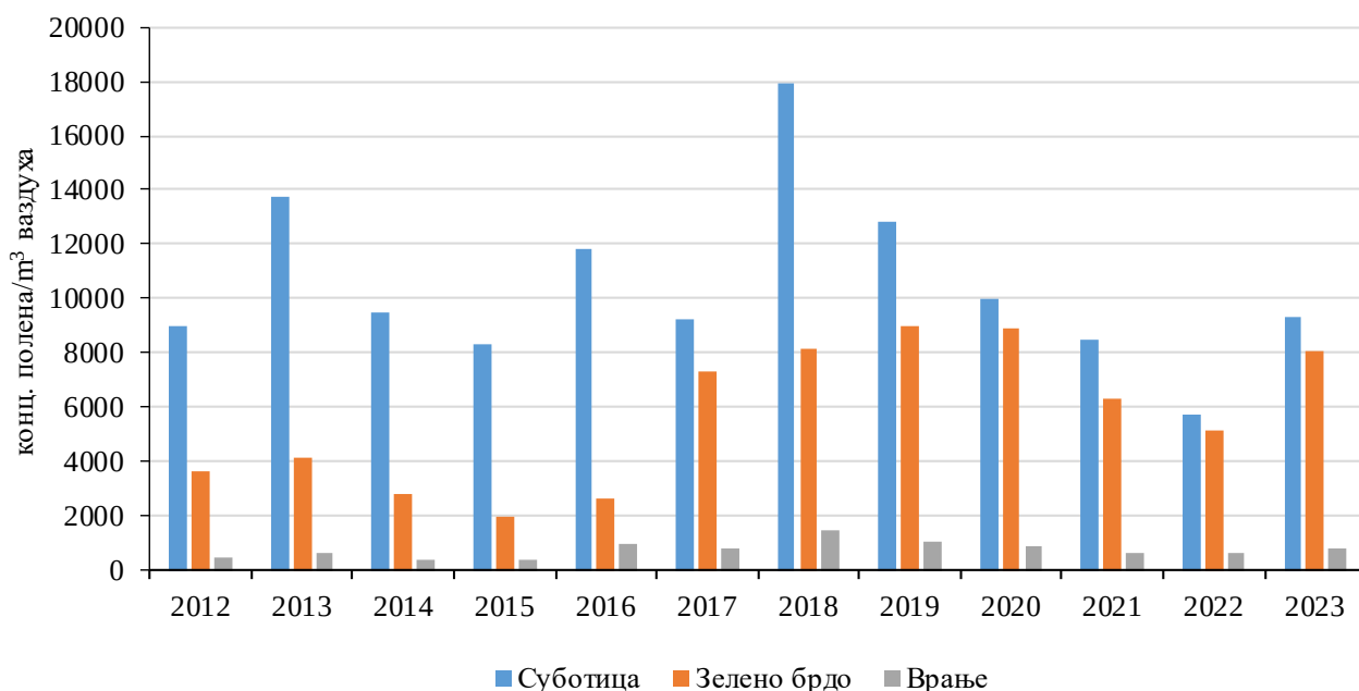
Слика 3.3.7. Просторна расподела укупне количине поленових зрна амброзије на три станице у Републици Србији у периоду 2012-2023. године
