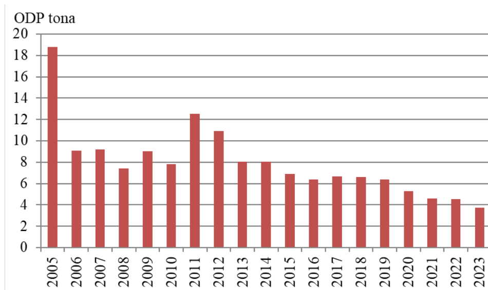
Слика 3.3.18. Потрошња супстанци које оштећују озонски омотач, у периоду 2005-2023. година
