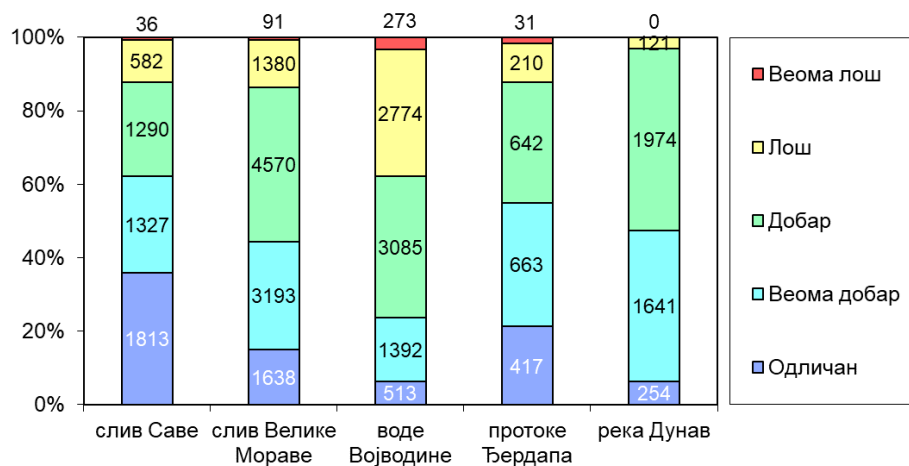
Слика 3.1.39. Анализа узорака воде методом SWQI по сливним подручјима Републике Србије (1998-2022. године)
