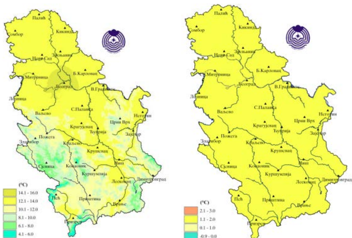
Слика 3.3.21. Расподела годишњих вредности температуре (°C) на подручју Републике Србије у 2023. години (лево) и одступања средње годишње температуре у (°C) од нормале 1991-2020. година (десно)
