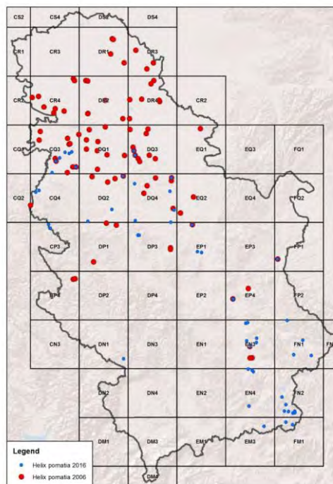
Слика 3.4.13. Карте откупних станица за све врсте лековитог биља (А), печурке (Б) и виноградарског пужа (В)
