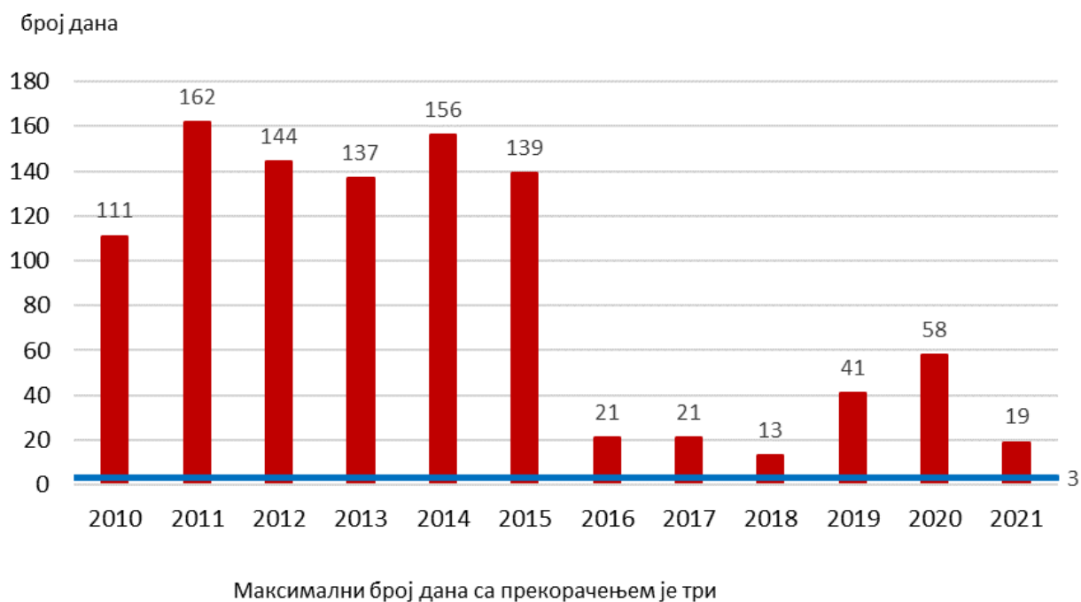
Слика 3.1.5. Број дана када је средња дневна вредност концентрације сумпор диоксида на станици Бор Градски парк прекорачила граничну вредност ( 125 \mu\text{g}/\text{m}^3 ) у периоду 2010-2021. године (дозвољен број дана је три током једне календарске године)
