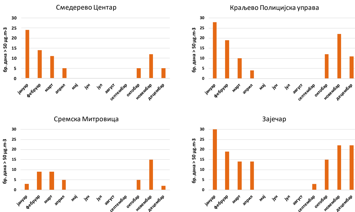
Слика 2.26. Приказ броја дана са прекорачењем дневне ГВ PM_{10} ( \mu g/m^3 ) по месецима 2020. године
