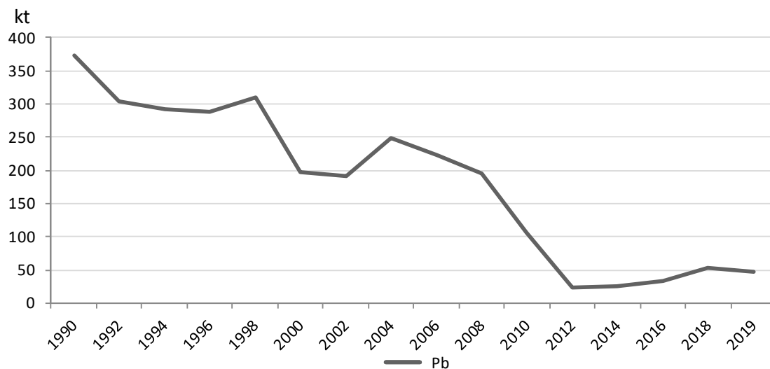
Слика 2.15. Емитоване количине Pb у Републици Србији у периоду 1990-2019. године
