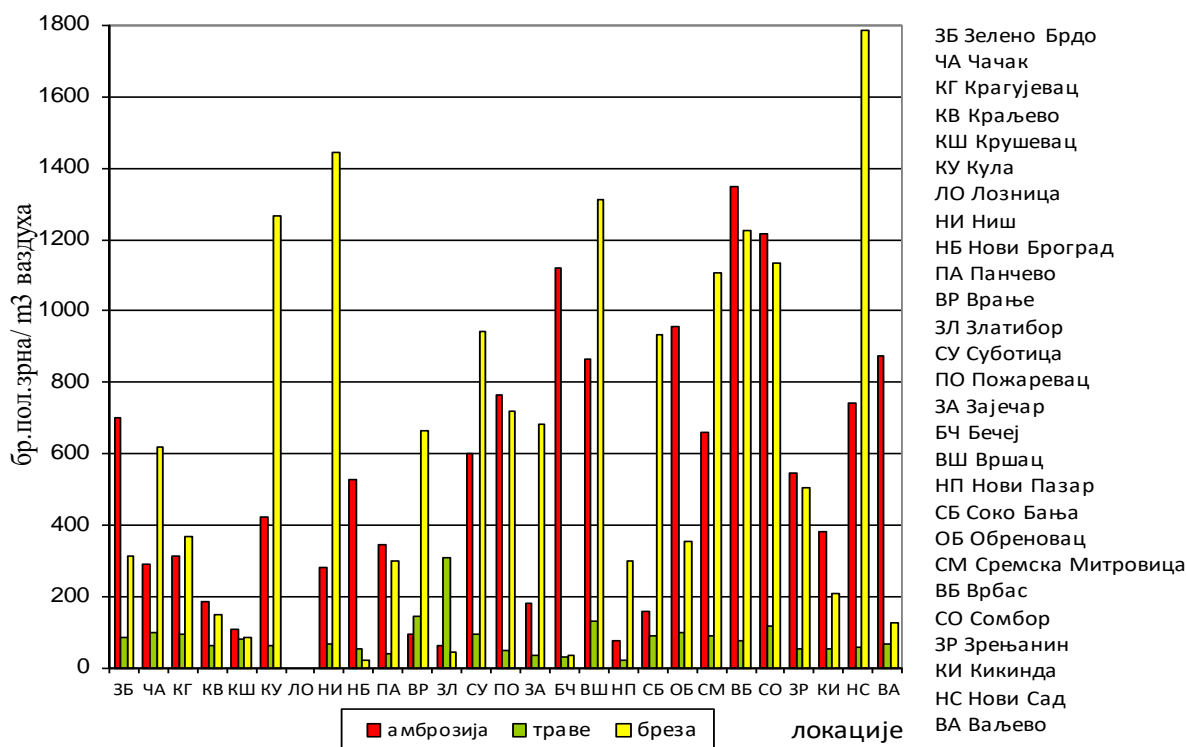
Слика 2.33. Максимална концентрација полених зрна на свим станицама у Републици Србији у 2020. години
