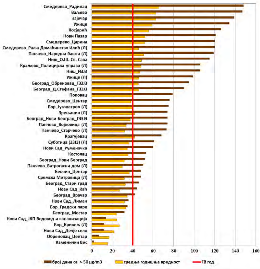
Слика 2.25. Упоредни приказ средње годишње концентрације PM_{10} ( \mu\text{g}/\text{m}^3 ) и броја дана са прекорачењем ГВ у 2020. години
