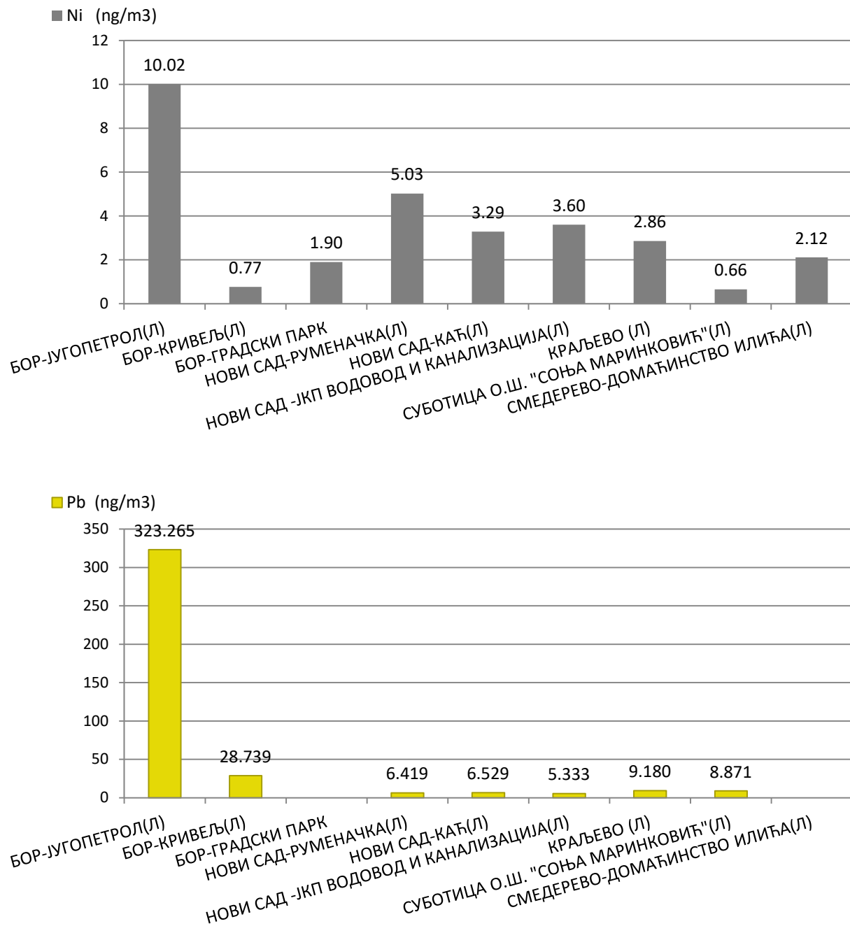
Слика 2.31. Садржај арсена, кадмијума, никла и олова у суспендованим честицама РМ 10
