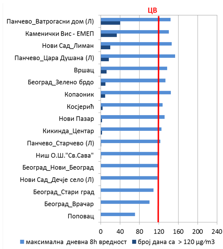
Слика 2.27. Упоредни приказ максималних дневних осмосатних концентрација O_3 ( \mu g/m^3 ) и броја дана са прекорачењем ЦВ у 2020. години
