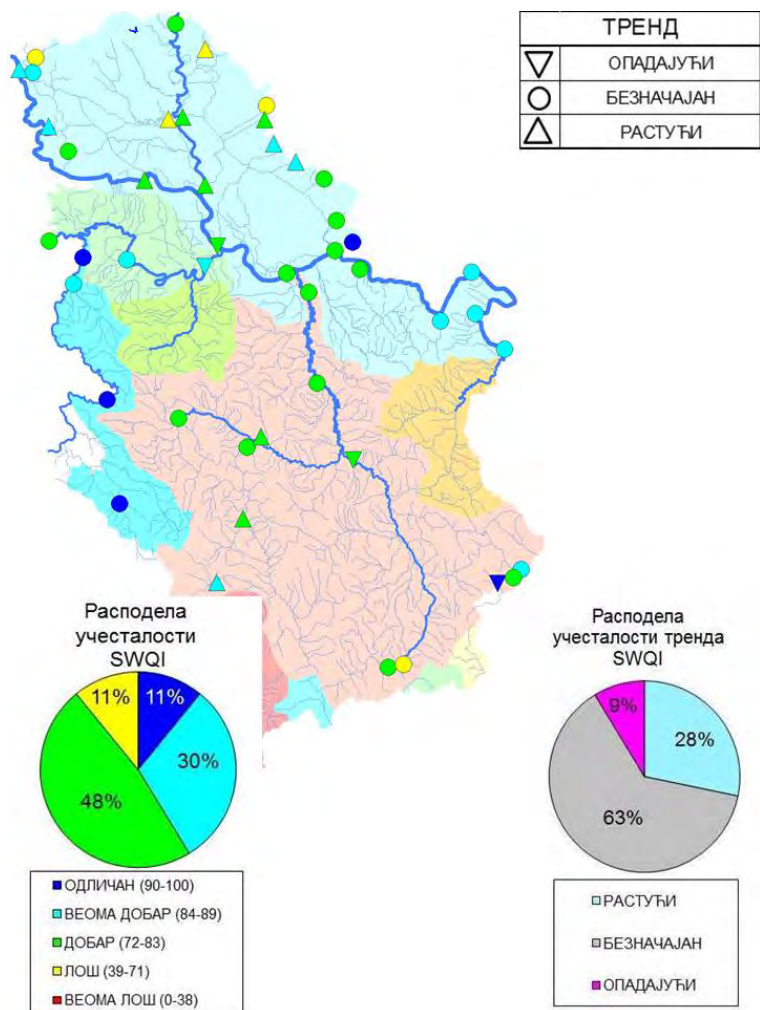
Слика 3.14. Тренд и средња вредња SWQI у водотоцима Републике Србије (2010-2019. године)
