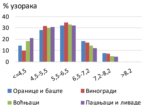
Слика 5.2. Супституционална киселост (pH у nKCl-y)
