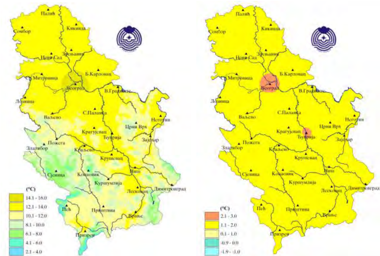
Слика 40. Распoдела годишњих вредности температуре (лево) на подручју Републике Србије у 2019. години и одступања средње годишње температуре у (°C) од нормале за период 1981-2010. године (десно)
