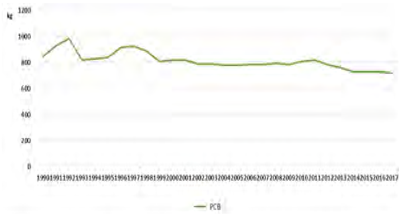
Слика 16. Емитоване количине полихлорованих бифенила у Републици Србији у периоду 1990-2017. године
