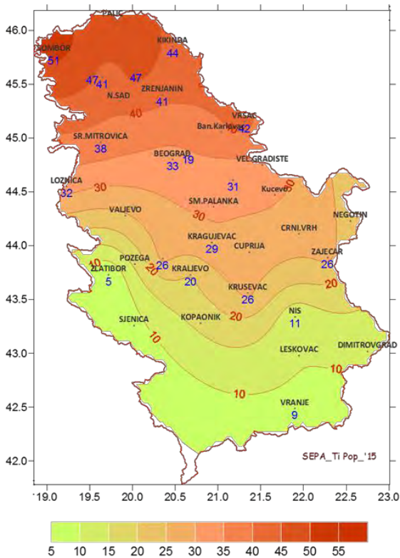
Слика 26. Географска расподела броја дана са прекорачењем граничне концентрације амброзије, 15, зрна/м 3 , током сезоне 2014.
