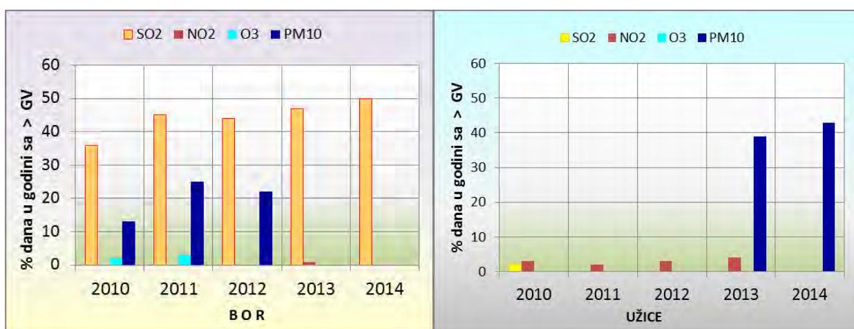
Слика 21. Процент дана током године са дневним концентрација SO_2 , NO_2 , O_3 и PM_{10} > ГВ у агломерацијама Бор и Ужице у периоду 2010 – 2014. године
