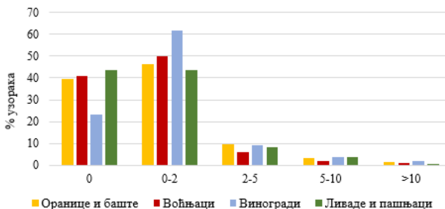
Слика 70. Садржај CaCO_3 (%)
