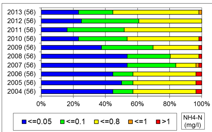
Слика 37. Расподела учесталости амонијума у водотоцима Републике Србије (2004-2013.)
