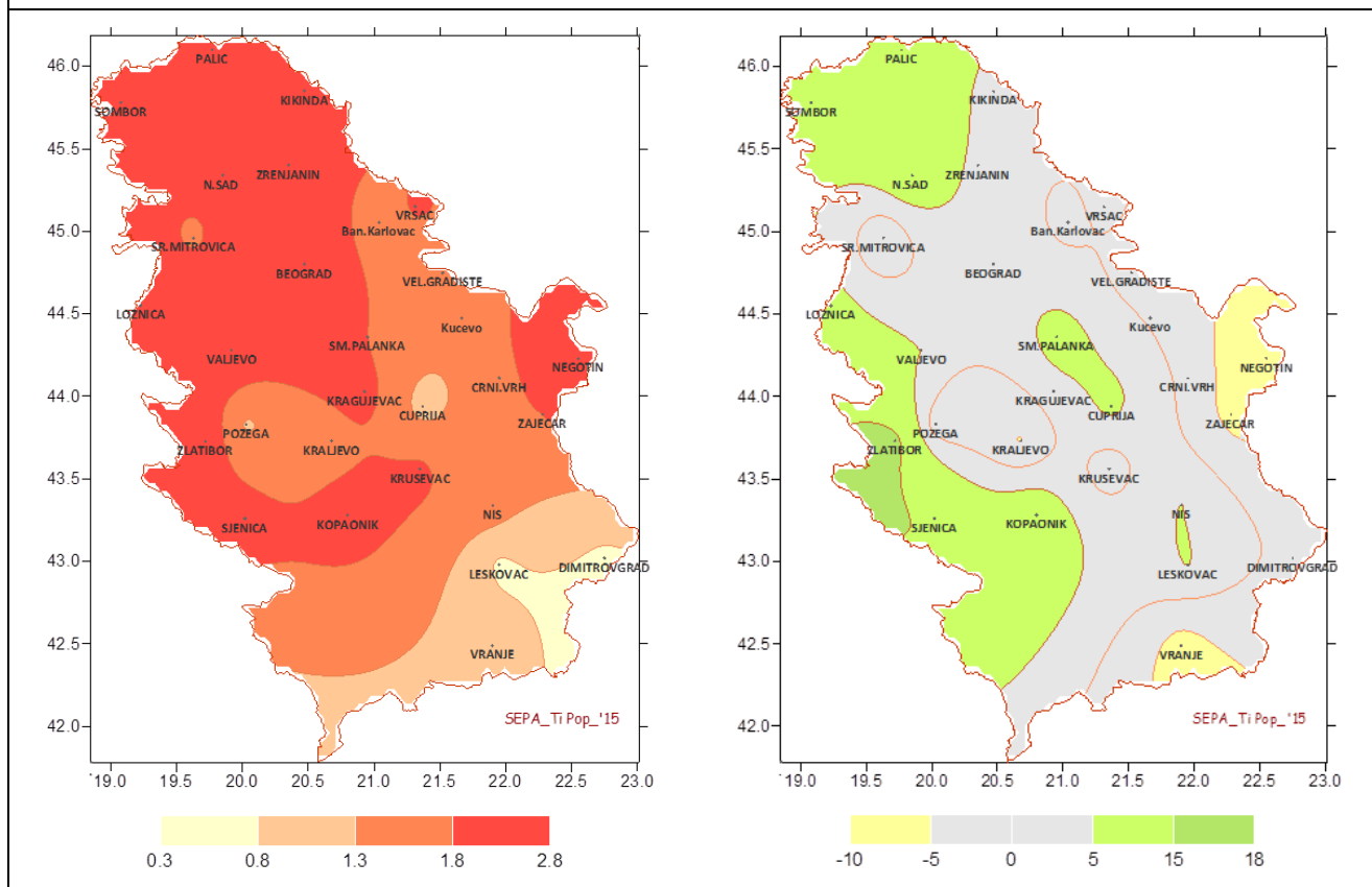
Слика 30. Географска расподела тренда годишњих вредности температуре и количина падавина на подручју Републике Србије у периоду 1951 – 2014; Лево - тренд годишњих температура ваздуха у °C/100 година Десно - тренд годишњих суме падавина у % N6190/50 година
