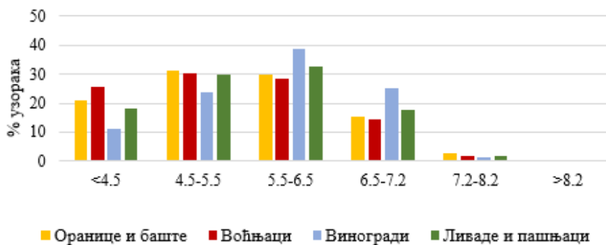
Слика 69. Супституционална киселост ( pH у KCl-y)
