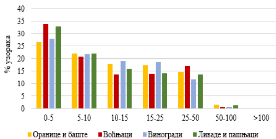
Слика 71. Садржај лакоприступачних облика фосфора ( P_2O_5 -mg/100g)
