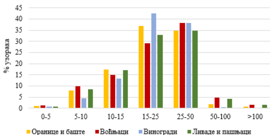
Слика 72. Садржај лакоприступачних облика калијума ( K_2O -mg/100g)
