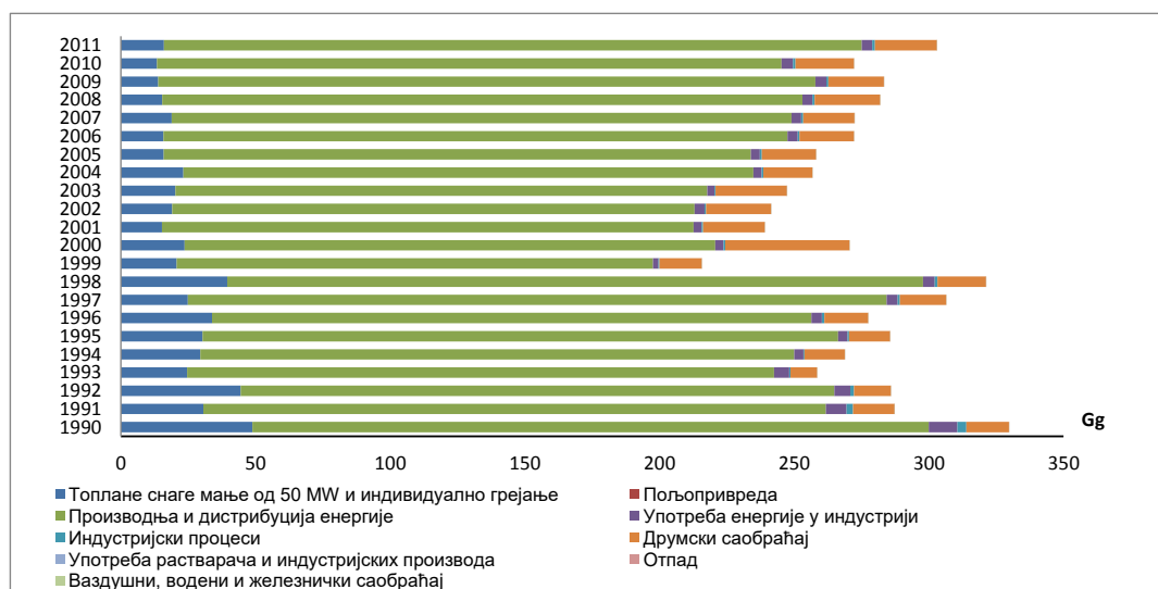
Слика 7. Емисије SO x у периоду од 1990. до 2011.године (Gg/год)
