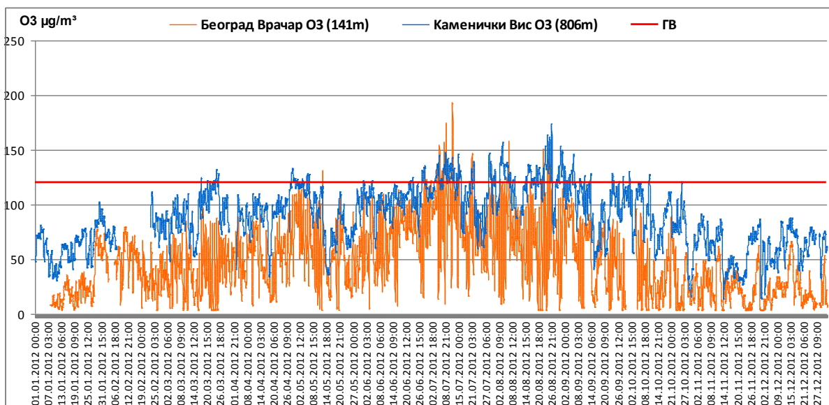
Слика 27. Годишњи ход 8-сатних концентрација приземног озона (О3) на станицама Београд_Врачар и Каменички Вис.
