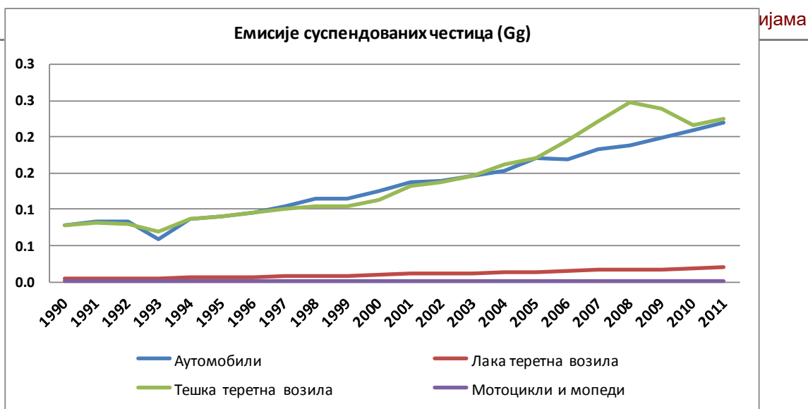
Слика 26. Емисије суспендованих честица (Gg) по категоријама
