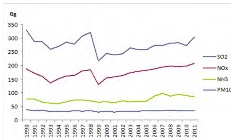
Слика 12. Емисије примарних суспендованих честица и секундарних прекурсора суспендованих честица (Gg/год)
