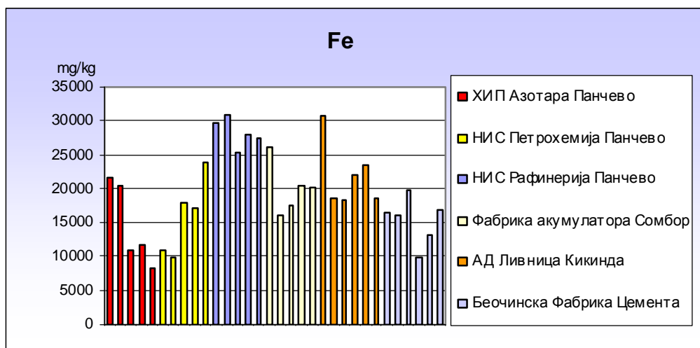
Слика 110. Fe у земљишту индустријских зона Војводине
