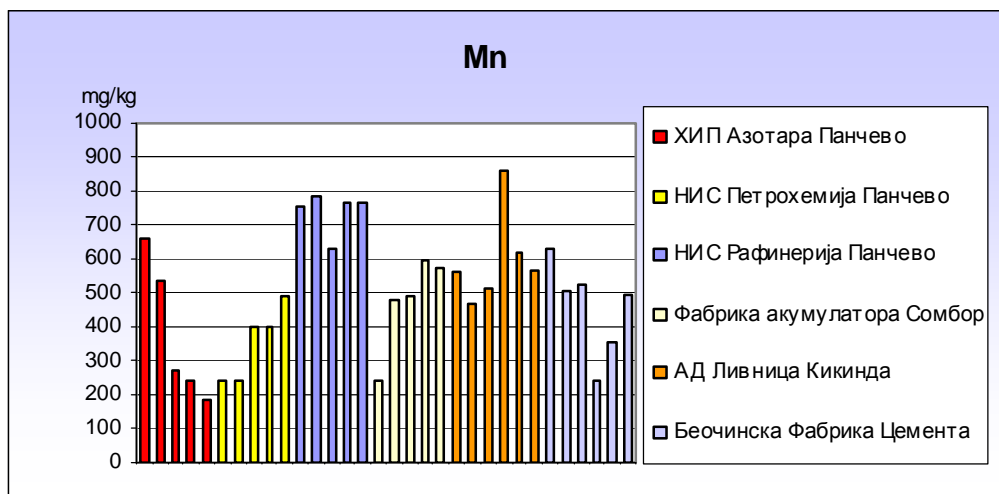
Слика 111. Mn у земљишту индустријских зона Војводине
