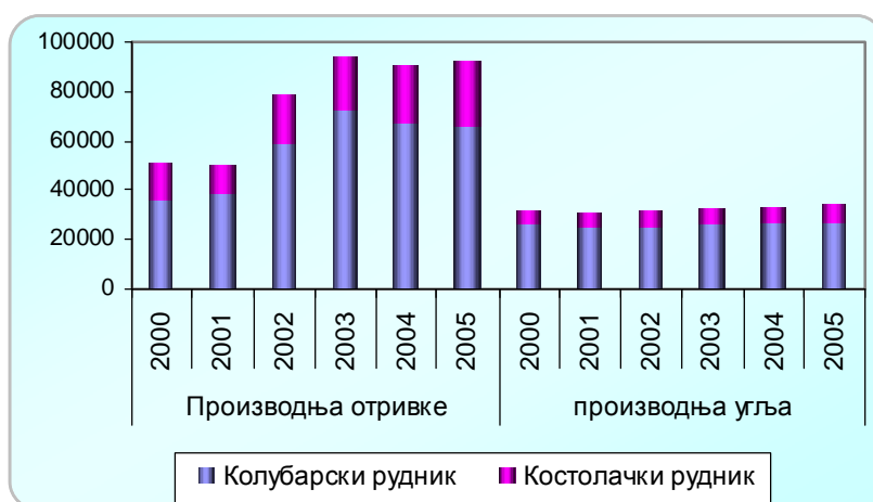
Слика 34. Производња угља и отривке
