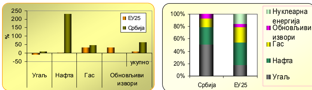
Промене у потрошњи укупне енергије и енергената ЕУ25 (период 1995-2003) и Србије (1994-2003) Учешће енергената у бруто потрошњи енергије 2003. године за ЕУ25 и Србију Слика 30. Парарелни приказ индикатора о потрошњи енергије и учешћу енергената за ЕУ25 и Србију
