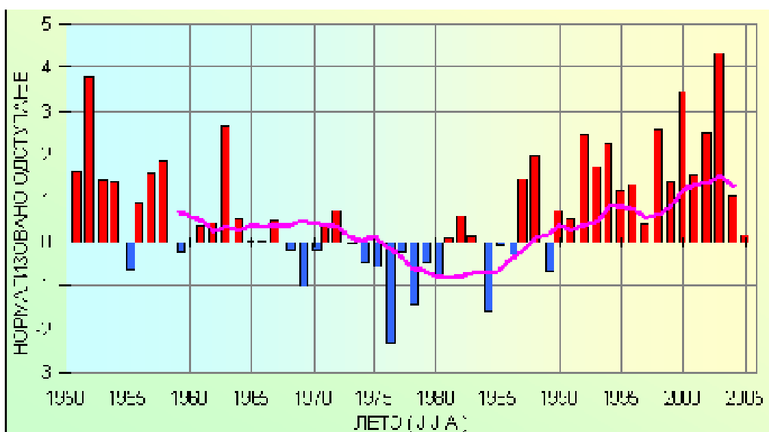
Слика 46. Нормализована одступања, са десетогодишњим клизним срењаком годишње (горе) и летње (доле) температуре ваздуха у Републици Србији, период 1951-2005.
