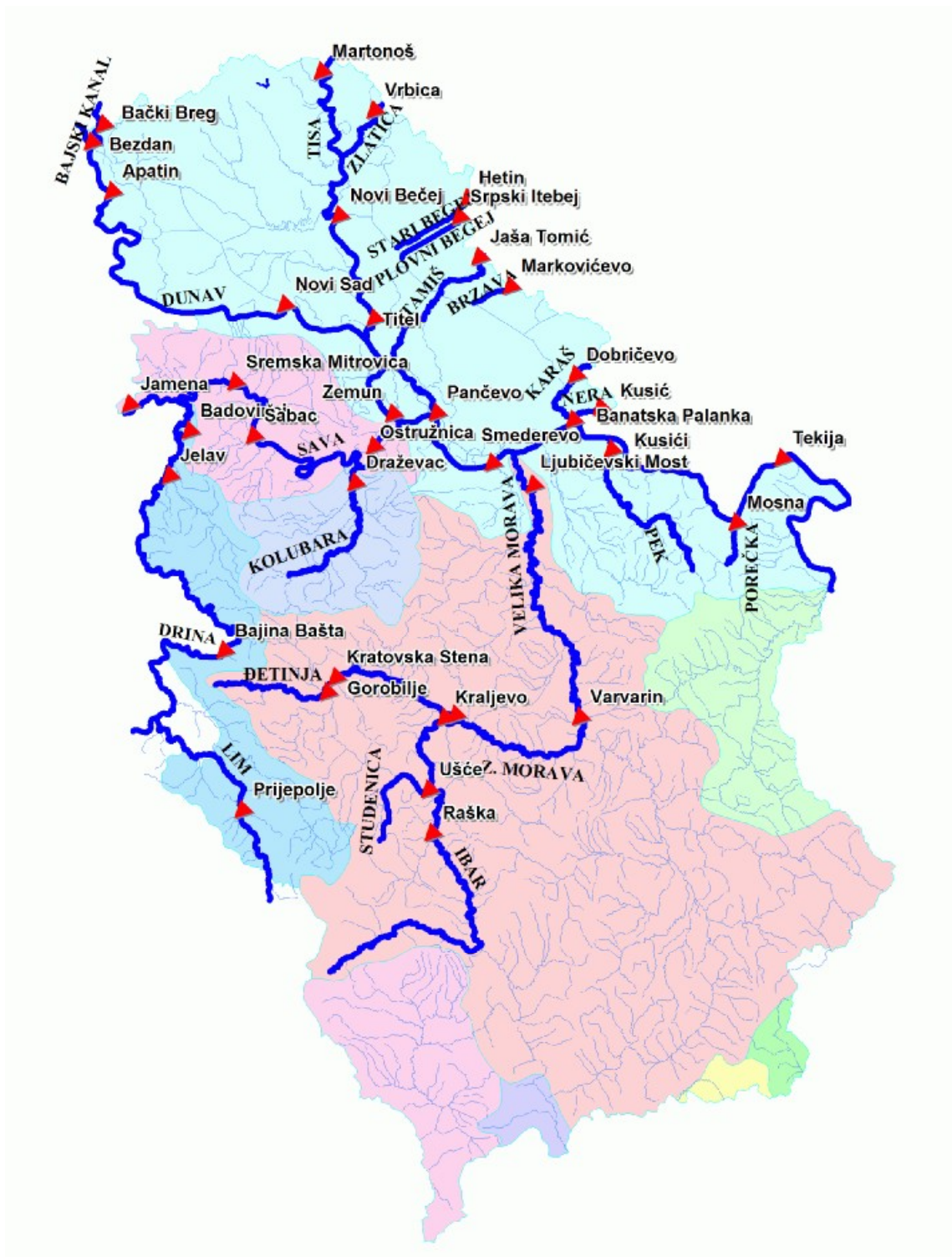
Слика 63. Карта профила коришћених у Извештају на којима испитивање квалитета површинских вода врши Републички хидрометеоролошки завод
