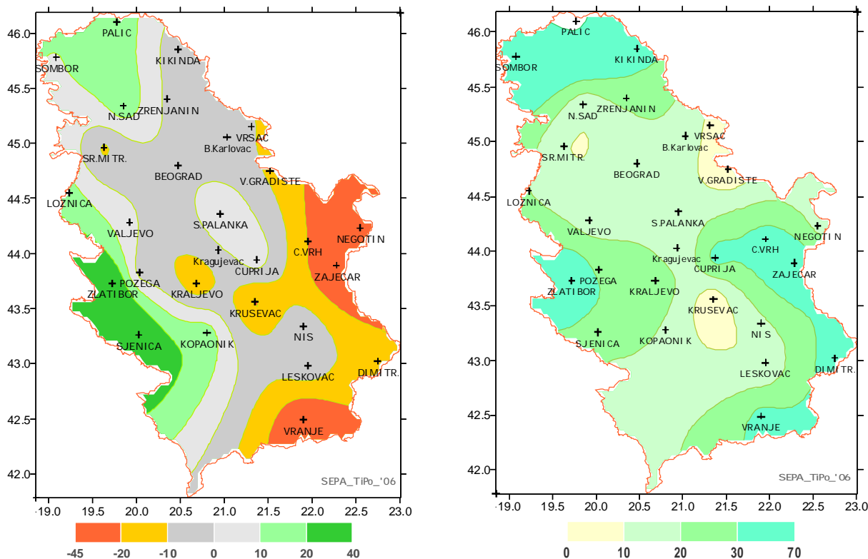
1951-2005. 1991-2005 Слика 49. Тренд годишњих сума падавина на подручју Србије; лево 1951-2005, у % Н1961-1990 за 50 година, десно 1991-2005, у % Н1961-1990 за 15 година
