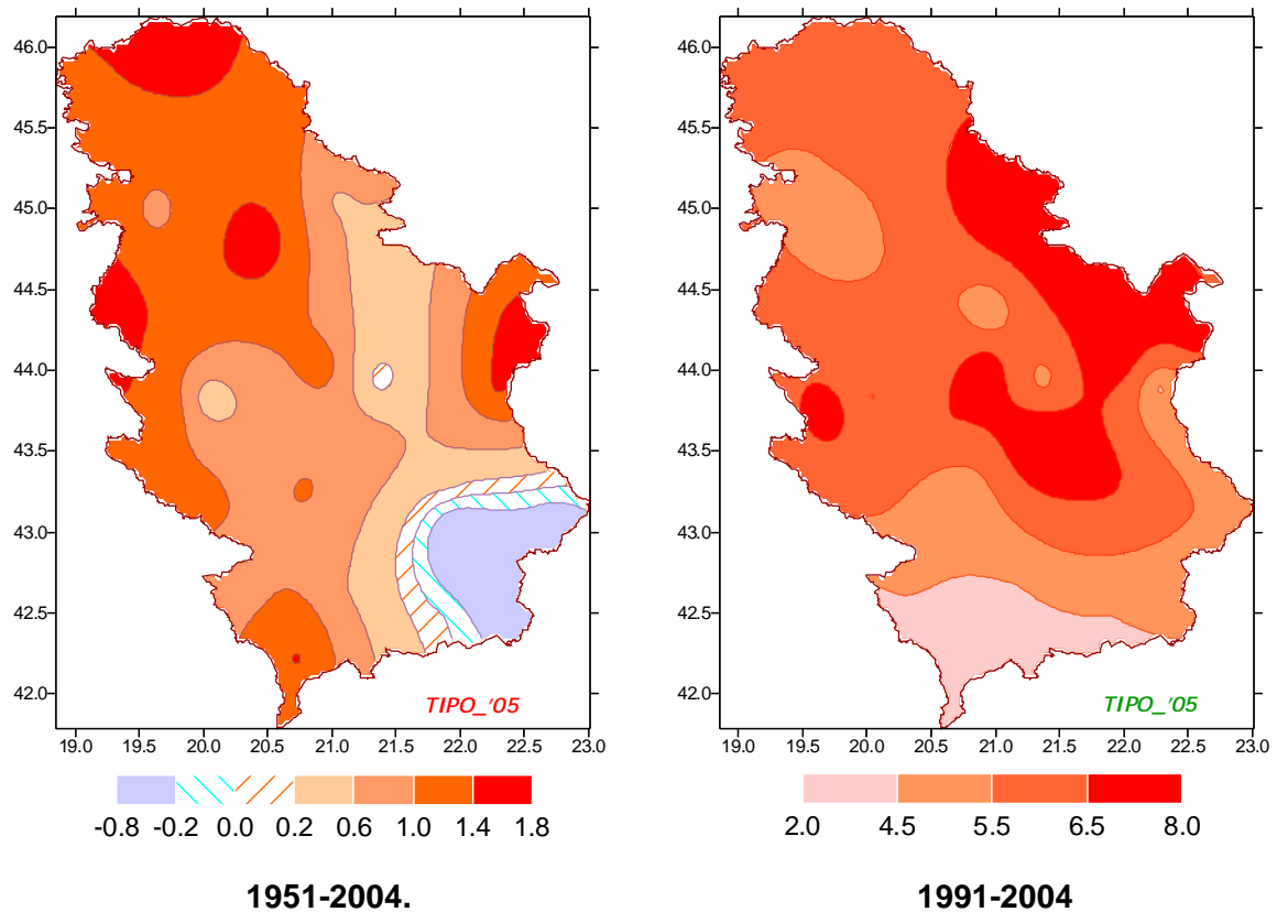
Слика 28. Територијална расподела тренда годишње температуре ваздуха на подручју Србије. Скала је изражена у ^{\circ}\text{C}/100 година
