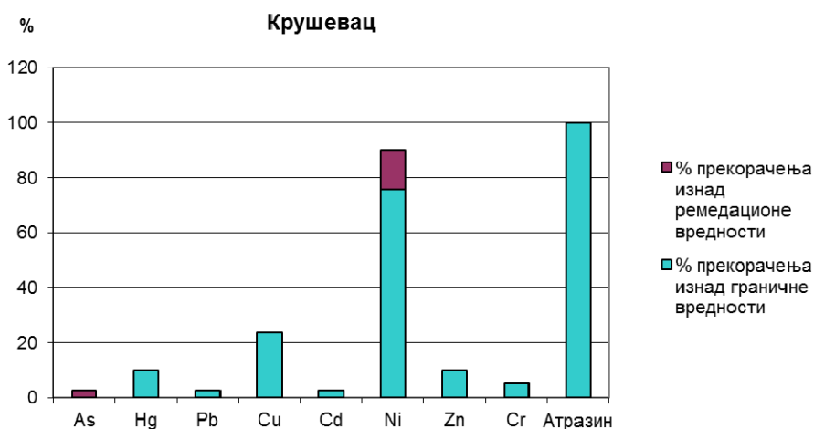
Слика 4. Процент прекорачења граничних и ремедиационих вредности
