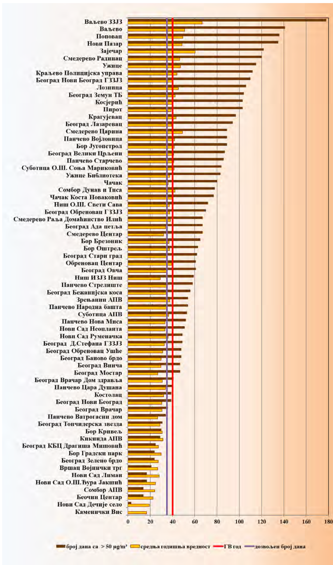
Слика 13. Упоредни приказ средње годишње концентрације \text{PM}_{10} ( \mu\text{g}/\text{m}^3 ) и броја дана са прекорачењем ГВ у 2022. години
