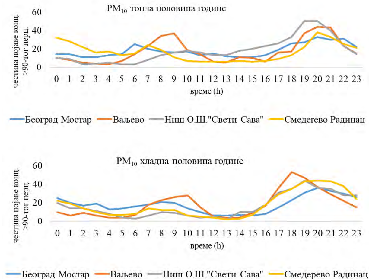
Слика 31. Суспендоване честице PM 10 - честина појаве концентрација већих од 90-тог перцентила током дана, у топлој и хладној половини године
