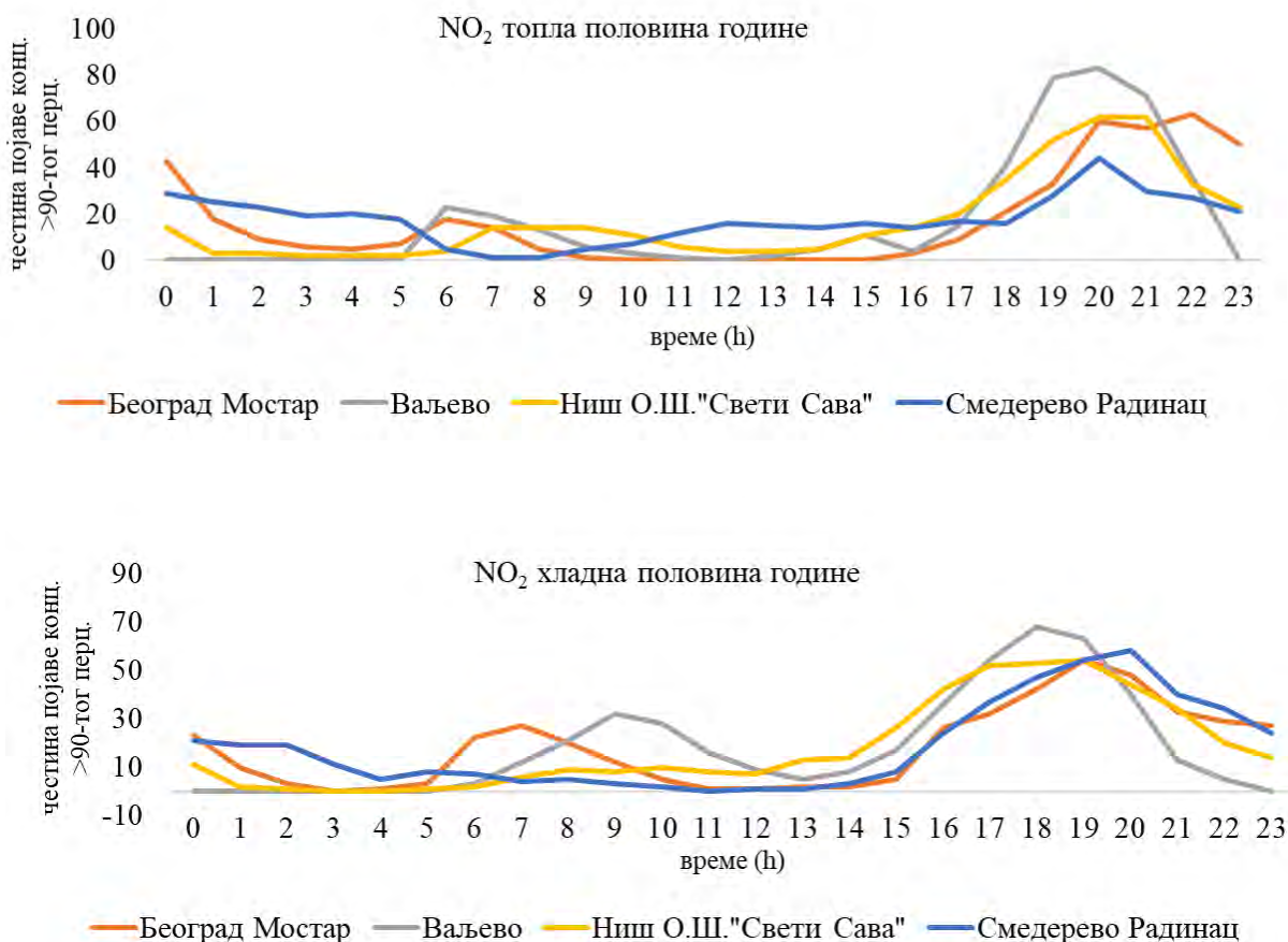
Слика 28. Азот диоксид - честина појаве концентрација већих од 90-тог перцентиала током дана, у топлој и хладној половини године
