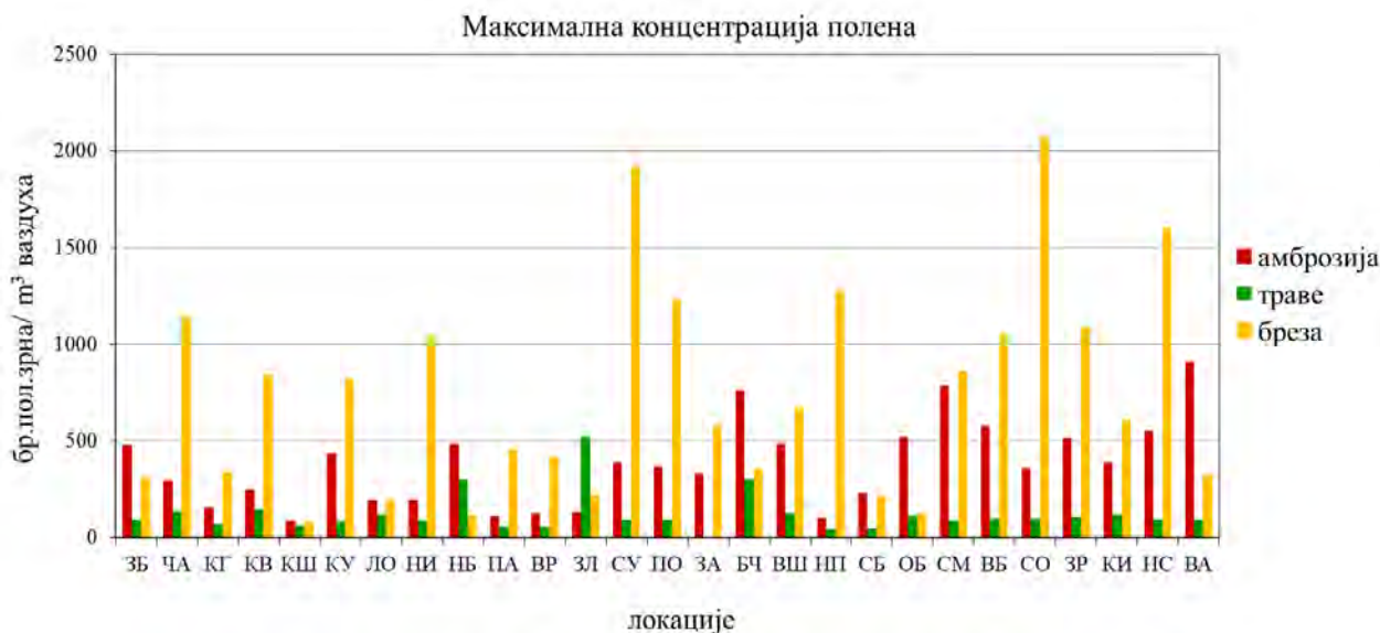
Слика 41. Максимална концентрација полевих зрна на свим станицама у Републици Србији у 2022. години
