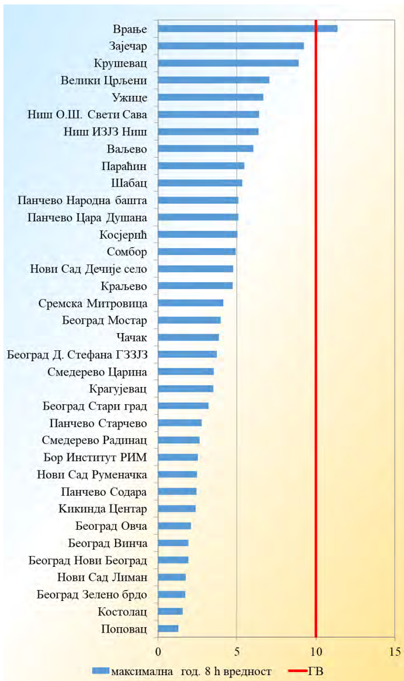
Слика 17. Приказ максималне осмосатне концентрације CO ( \text{mg}/\text{m}^3 ) у 2022. години
