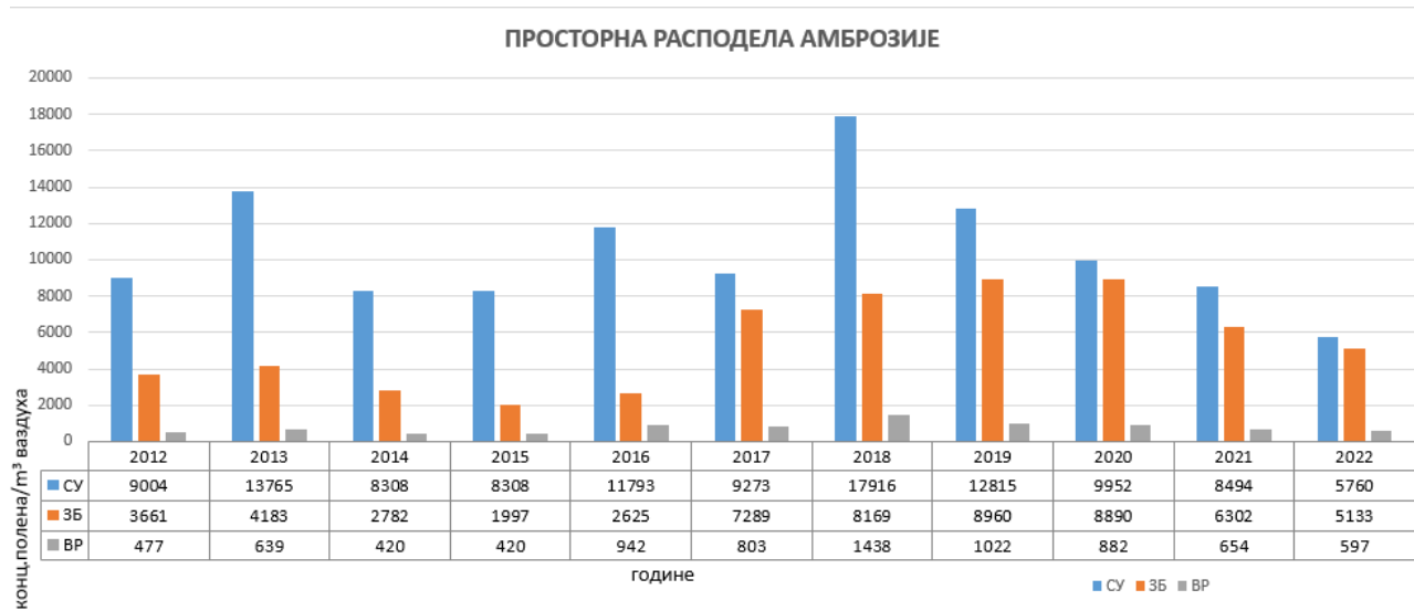
Слика 46. Просторна расподела укупне количине поленових зрна амброзије на три станице у Републици Србији у периоду 2012-2022. године
