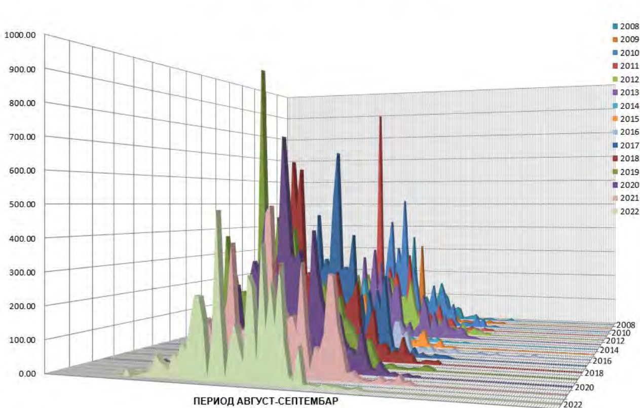
Слика 45. Емитовање полена амброзије у августу и септембру за период 2009-2022. године
