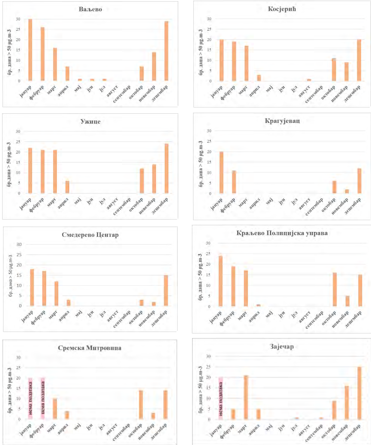
Слика 8. Приказ броја дана са прекорачењем дневне ГВ PM_{10} ( \mu g/m^3 ) по месецима у 2019. години
