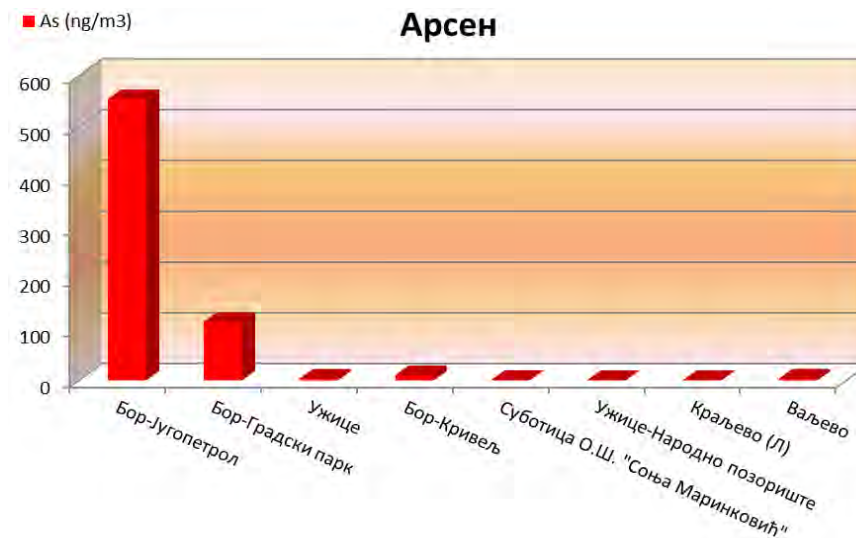
Слика 9. Средња годишња вредност арсена у 2019. години
