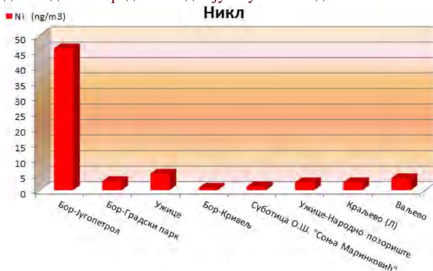
Слика 11. Средња годишња вредност никла у 2019. години
