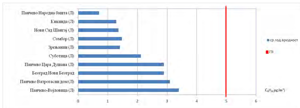
Слика 14. Приказ средње годишње концентрације бензена ( \mu\text{g}/\text{m}^3 ) у 2019. години
