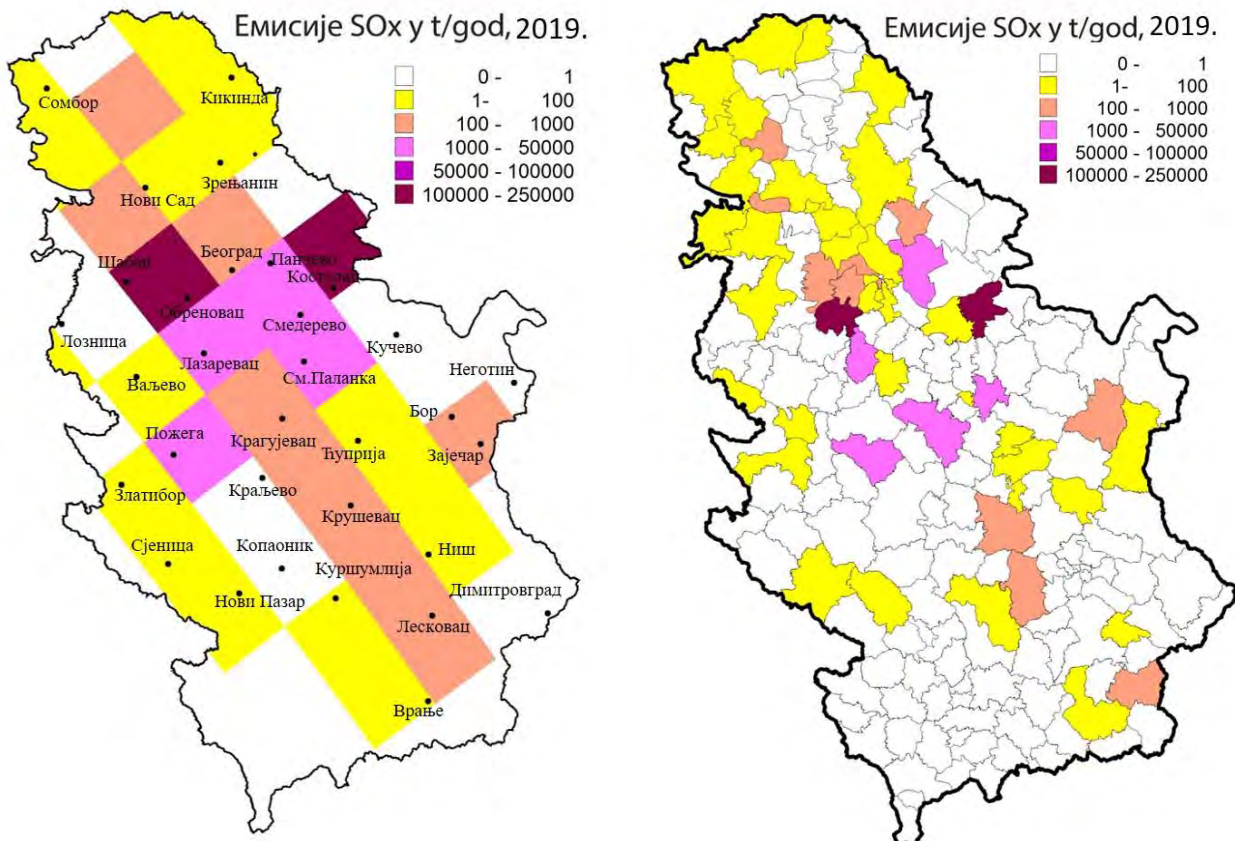
Слика 3. Просторна расподела емисија оксида сумпора, у t/год, током 2019. године у мрежи квадраната 50x50km (лево) и по општинама (десно)
