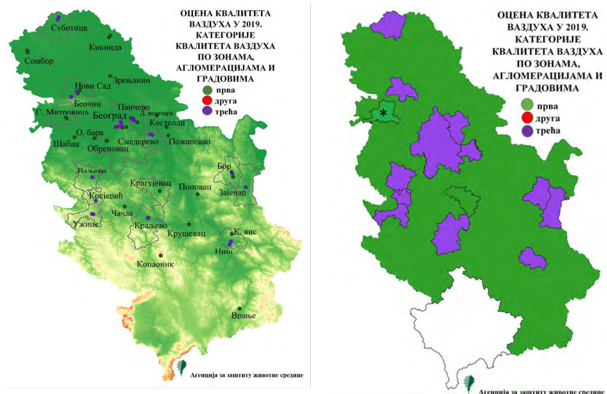
Слика 18. Категорије квалитета ваздуха 2019. године
