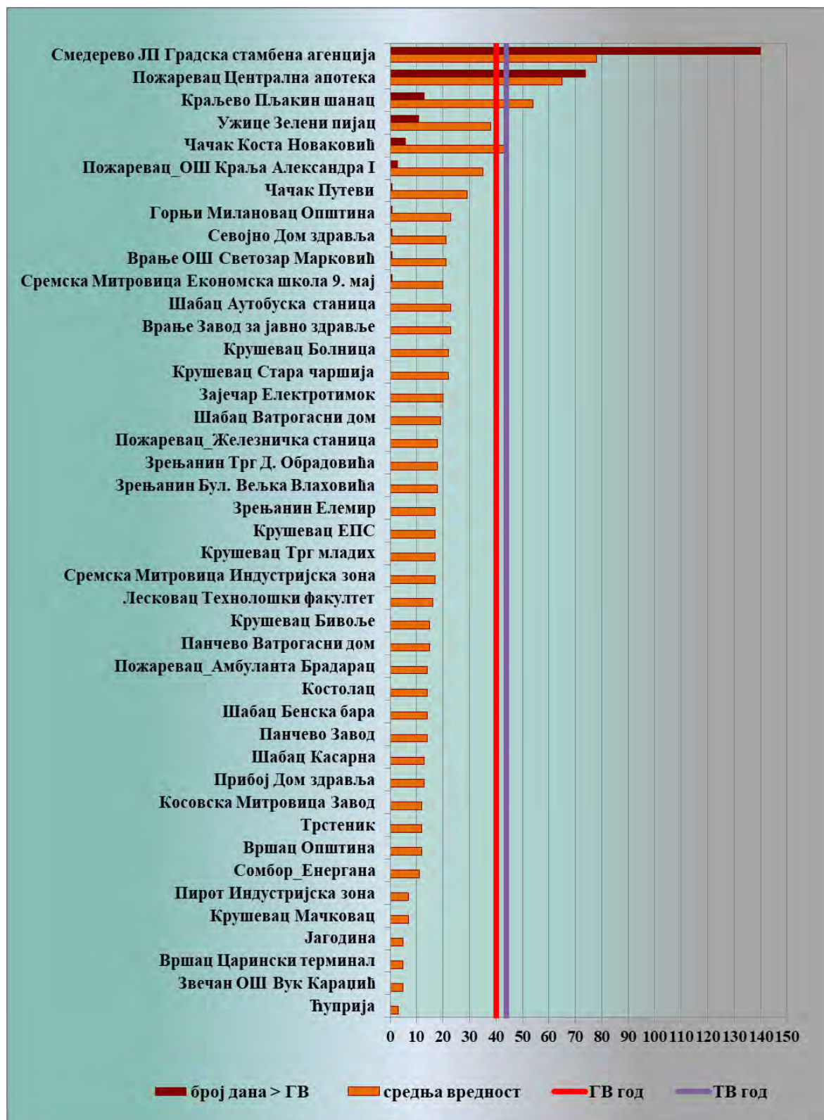
Слика 25. Средња годишња концентрација NO 2 (µg/m 3 ) и број дана са прекорачењем ГВ у 2019. години
