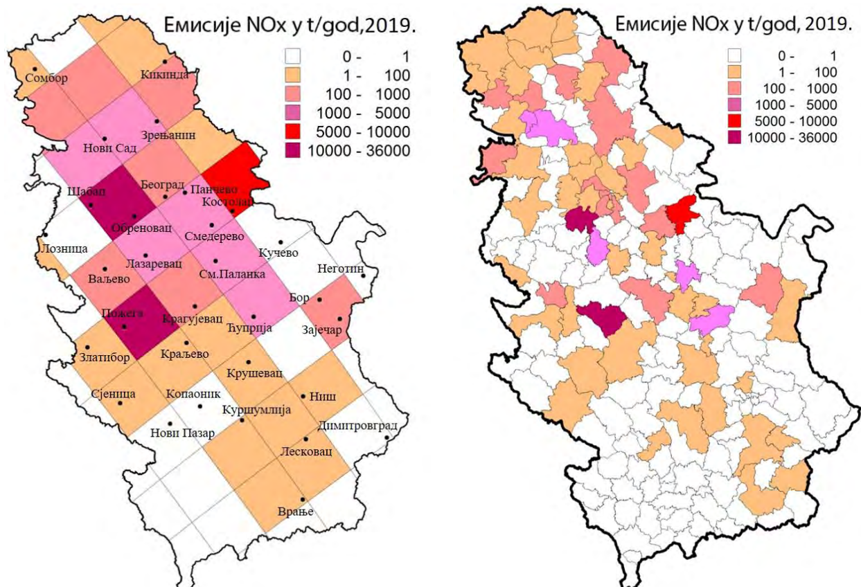
Слика 4. Просторна расподела емисија оксида азота током 2019. године (t/год.) у мрежи квадраната 50x50km (лево) и по општинама (десно)
