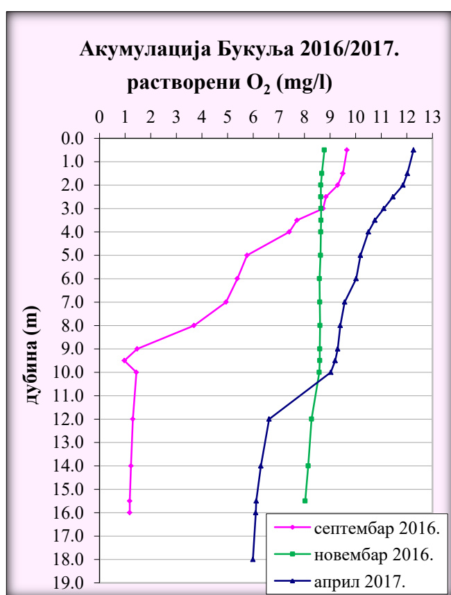
График 3.2.3.1. Распоред температуре воде и раствореног кисеоника по дубини акумулација, на локалитету А 1 (код бране)
