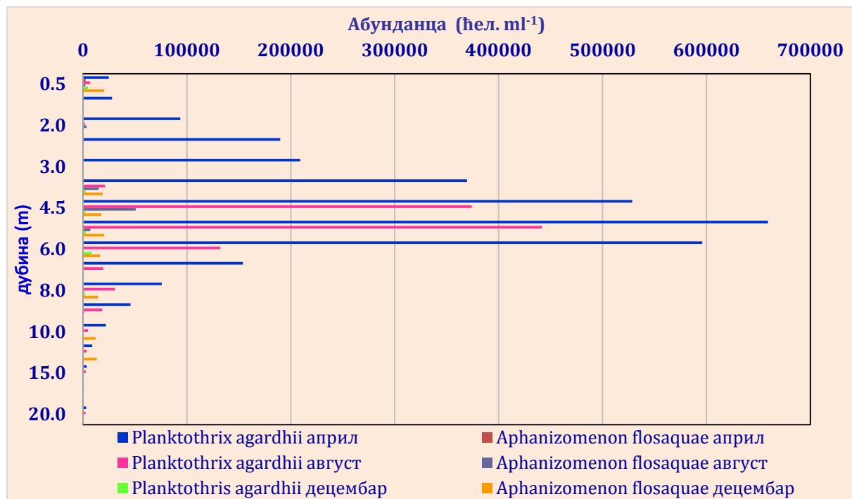
График 3.2.3.4. Абунданце доминантне ( Planktothrix agardhii ) и субдоминантне врсте ( Aphanizomenon flosaquae ) цијанобактерија по дубини акумулације Гараша, на локалитету А 1 2016. године
