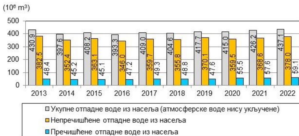
Слика 3.2.26. Количине отпадних вода у Републици Србији (2013-2022. године)
