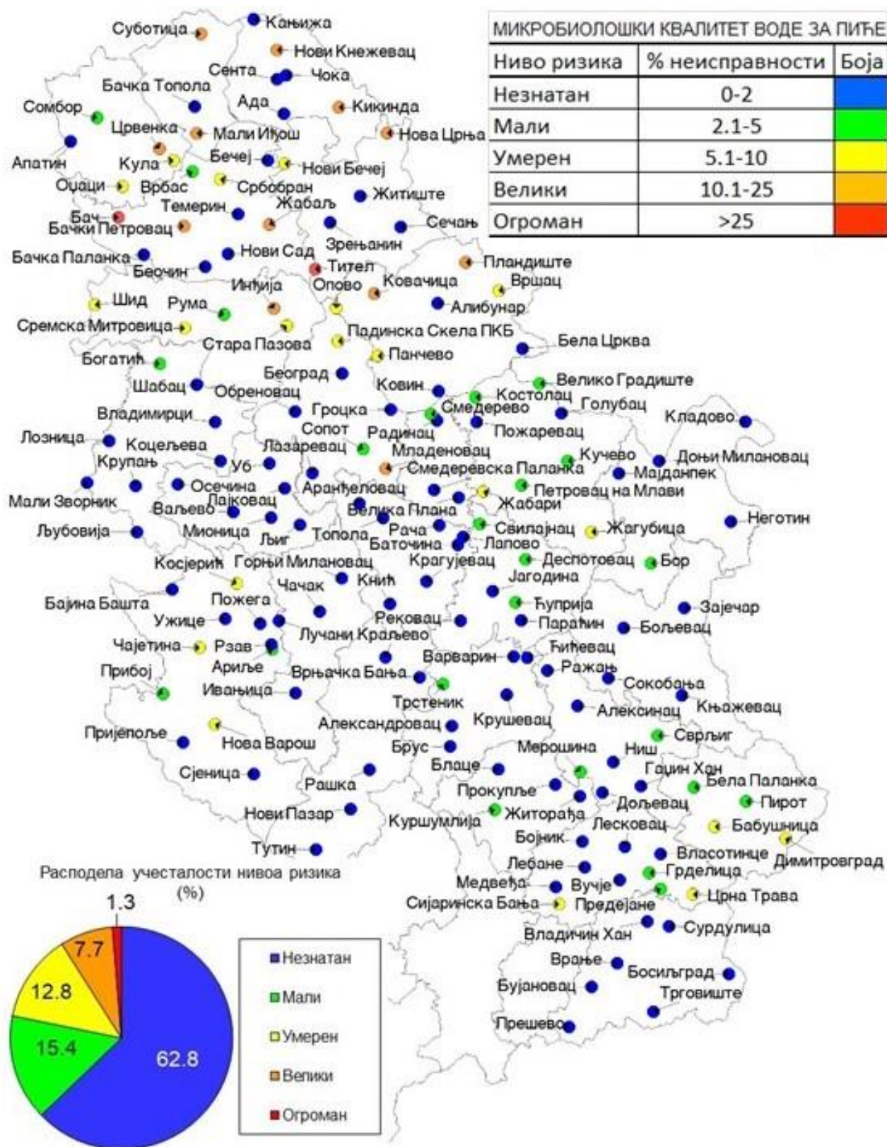
Слика 3.3.4. Микробиолошка неисправност воде за пиће јавних водовода градских насеља у 2022. години
