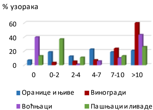
Слика 3.1.59. Садржај CaCO 3 (%)
