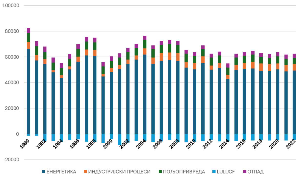
Слика 3.2.19. Укупне емисије гасова са ефектом стаклене баште са понорима, по секторима (kt)
