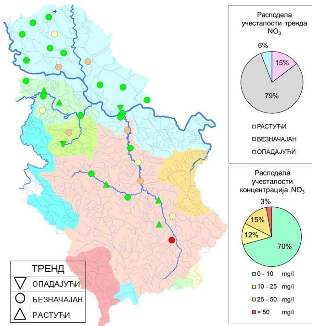
Слика 3.1.41. Тренд и средња вредња концентрација нитрата у подземним водама Републике Србије (2013-2022. године)
