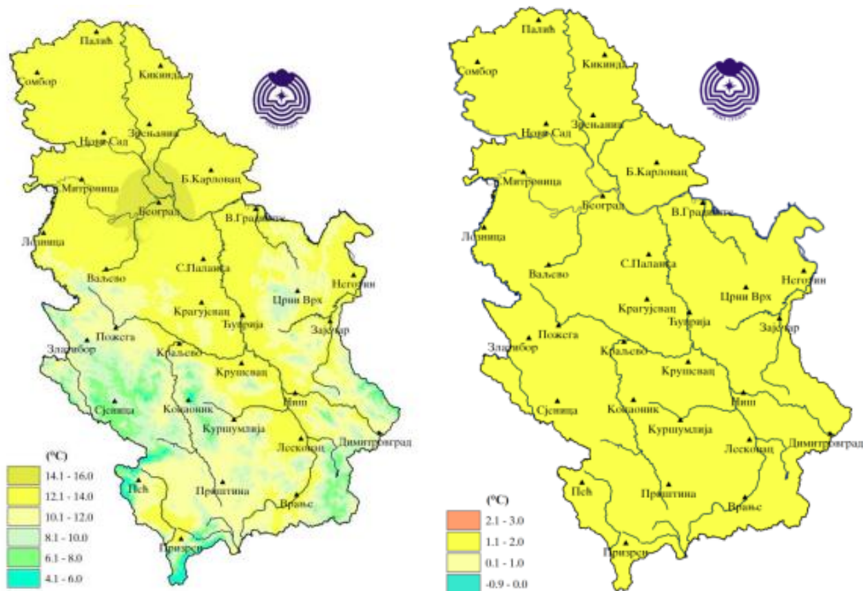
Слика 3.3.21. Распдела годишњих вредности температуре (°С) на подручју Републике Србије у 2023. години (лево) и одступања средње годишње температуре у (°С) од нормале 1991-2020. година (десно)
