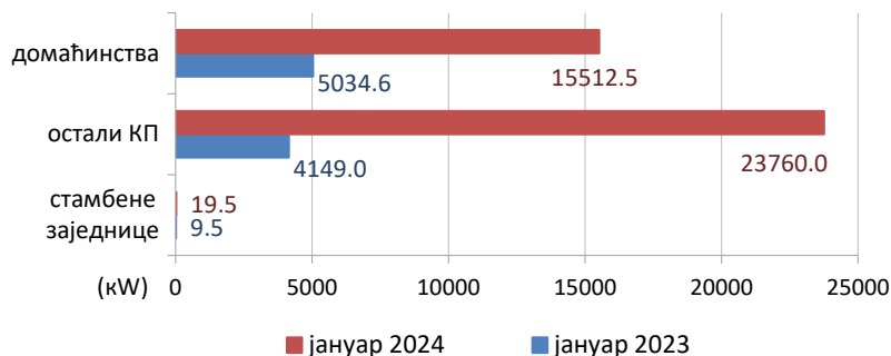
Слика 3.5.52. Укупна инсталисана снага у кВ по категоријама купаца-произвођача
